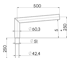
CROSSE SIMPLE
