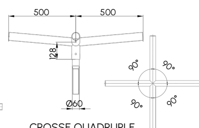
CROSSE QUADRUPLE
