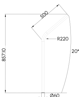
CROSSE MURALE 20°
